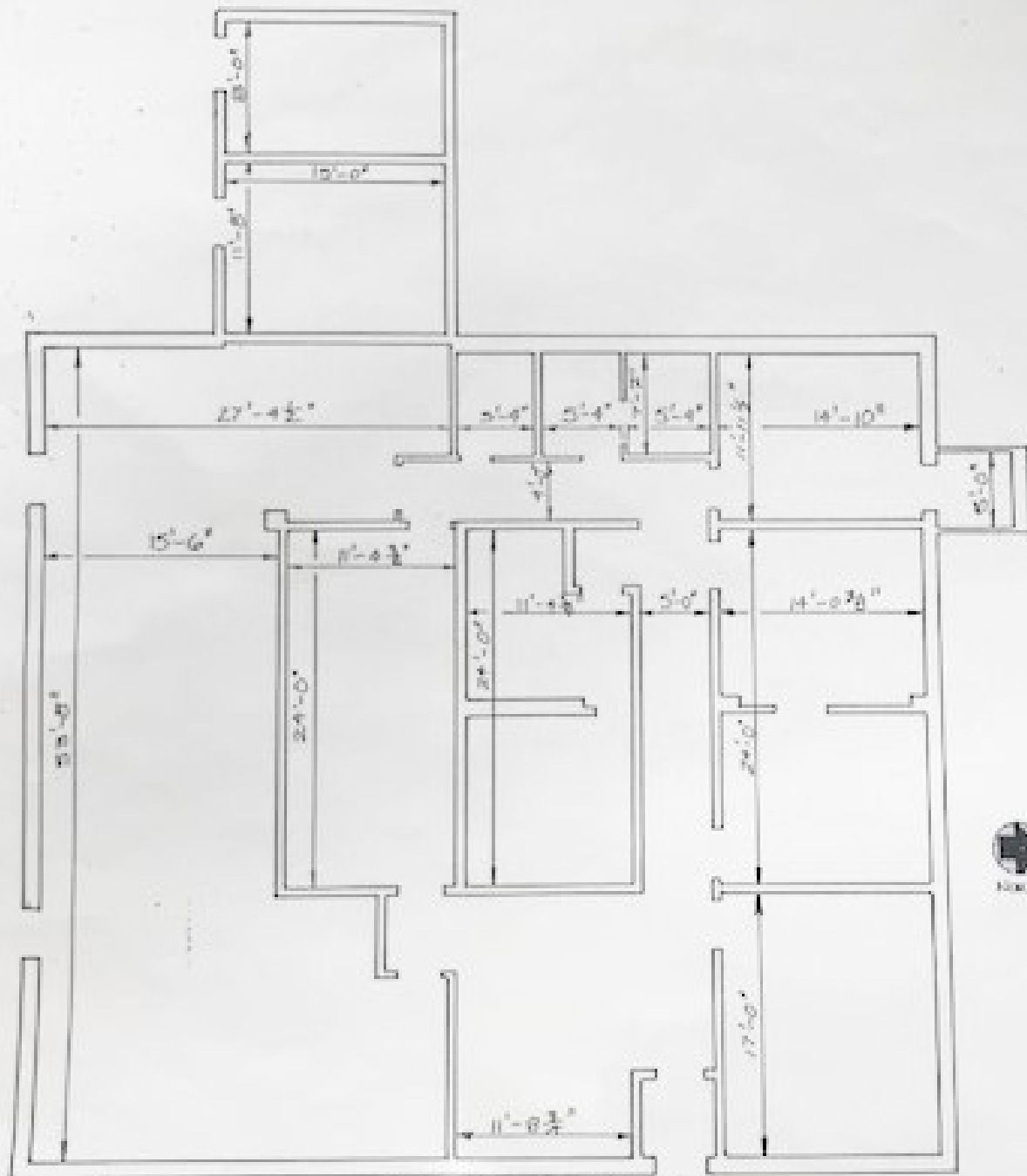
FLOOR PLAN - BLDG. 501 N.T.S.
